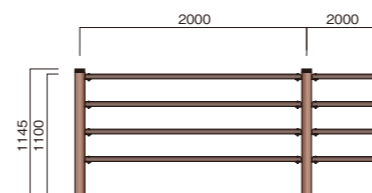
FB-4B1120C 重量:12.9kg/m 支柱:10.6kg/本 FB-4B1120W 重量:12.3kg/m 支柱:9.4kg/本
