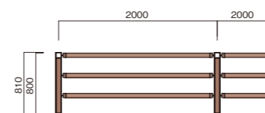
FA-3B0820C 重量:18.0kg/m 支柱:15.9kg/本 FA-3B0820W 重量:16.9kg/m 支柱:13.6kg/本
