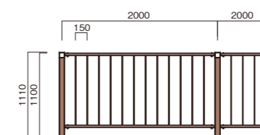
FA-K1120C 重量:19.7kg/m 支柱:20.3kg/本 FA-K1120W 重量:18.2kg/m 支柱:17.4kg/本
