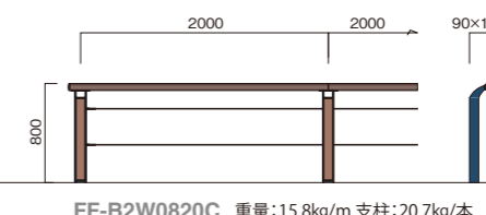
FF-B2W0820C 重量:15.8kg/m 支柱:20.7kg/本 FF-B2W0820W 重量:14.9kg/m 支柱:18.9kg/本
