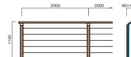
FF-B5W1120C 重量:20.7kg/m 支柱:24.5kg/本 FF-B5W1120W 重量:19.3kg/m 支柱:21.7kg/本
