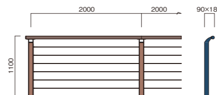
FF-B6W1120C 重量:21.7kg/m 支柱:24.5kg/本 FF-B6W1120W 重量:20.3kg/m 支柱:21.7kg/本
