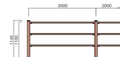
FB-3B1120C 重量:11.0kg/m 支柱:10.6kg/本 FB-3B1120W 重量:10.4kg/m 支柱:9.4kg/本
