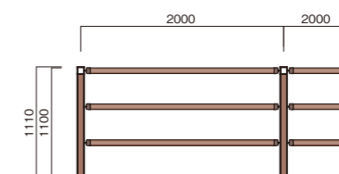
FA-3B1120C 重量:20.2kg/m 支柱:20.3kg/本 FA-3B1120W 重量:18.8kg/m 支柱:17.4kg/本
