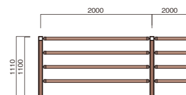
FA-4B1120C 重量:23.6kg/m 支柱:20.3kg/本 FA-4B1120W 重量:22.1kg/m 支柱:17.4kg/本
