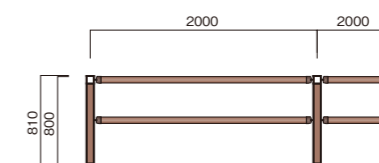
FA-2B0820C 重量:14.7kg/m 支柱:15.9kg/本 FA-2B0820W 重量:13.5kg/m 支柱:13.6kg/本
