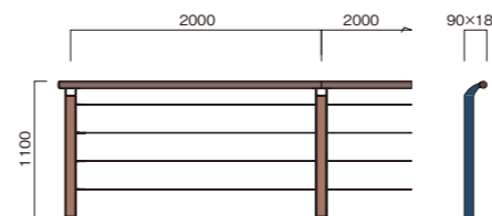
FF-B4W1120C 重量:19.7kg/m 支柱:24.5kg/本 FF-B4W1120W 重量:18.3kg/m 支柱:21.7kg/本
