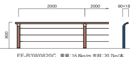
FF-B3W0820C 重量:16.8kg/m 支柱:20.7kg/本 FF-B3W0820W 重量:15.9kg/m 支柱:18.9kg/本
