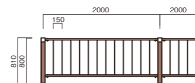
FA-K0820C 重量:15.5kg/m 支柱:15.9kg/本 FA-K0820W 重量:14.4kg/m 支柱:13.6kg/本
