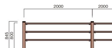
FB-3B0820C 重量:10.0kg/m 支柱:8.6kg/本 FB-3B0820W 重量:9.5kg/m 支柱:7.6kg/本
