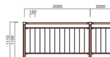
FA-BK1120C 重量:22.0kg/m 支柱:20.3kg/本 FA-BK1120W 重量:20.5kg/m 支柱:17.4kg/本
