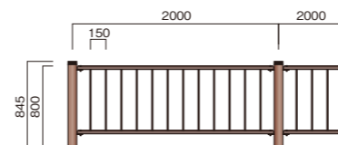
FB-K0820C 重量:11.8kg/m 支柱:8.6kg/本 FB-K0820W 重量:11.3kg/m 支柱:7.6kg/本
