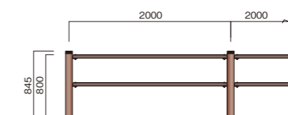
FB-2B0820C 重量:8.1kg/m 支柱:8.6kg/本 FB-2B0820W 重量:7.6kg/m 支柱:7.6kg/本
