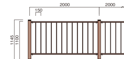
FB-K1120C 重量:14.8kg/m 支柱:10.6kg/本 FB-K1120W 重量:14.2kg/m 支柱:9.4kg/本
