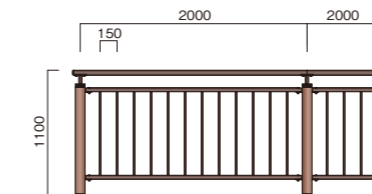
FB-BK1120C 重量:17.4kg/m 支柱:9.9kg/本 FB-BK1120W 重量:16.7kg/m 支柱:8.6kg/本
